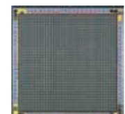
開発した37x37ピクセルの人工網膜チップ A 37x37 pixels artificial retina chip (3.2mmx3.2mm)
