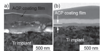
RFマグネトロンスパッタリング法により作製した非晶質リン酸カルシウム(ACP)薄膜(a)および家兎大腿骨埋入1週間後(b)の断面 Cross section of amorphous calcium phosphate (ACP) coating film fabricated by RF magnetron sputtering (a) before and (b) after 1 week implantation.
