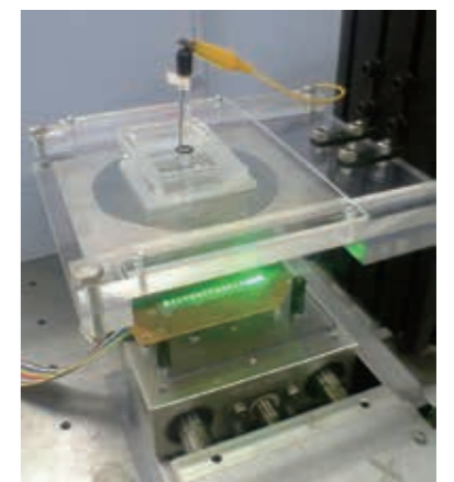
化学イメージングセンサシステムの外観 Chemical imaging sensor system
