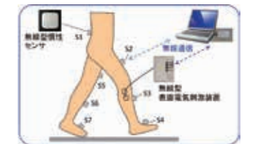
ウェアラブル運動計測システムの開発と運動機能評価への応用 Development of wearable motion measurement system and its application to evaluation of the motor function
