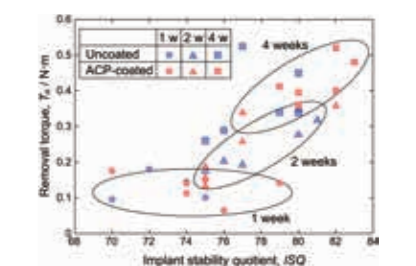
リン酸カルシウムコーティングを施したインプラントおよびコーティング無しインプラントの家兎大腿骨からの回転除去トルクとISQ値の関係 Relationship between ISQ and removal torque of ACP-coated and uncoated implants from the femur, 1, 2, and 4 weeks after implantation.
