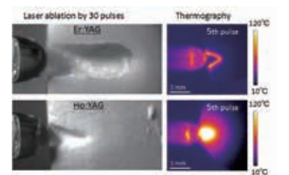
レーザーアブレーション中の熱画像 Thermal imaging during laser ablation
