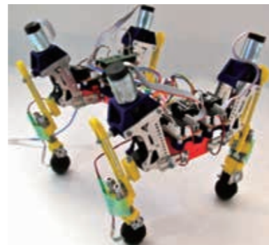
身体特性や移動速度の変化に応じて脚の動かし方を自己組織的に適応可能な4脚ロボット Quadruped robot driven by a fully decentralized neural network-based control.
