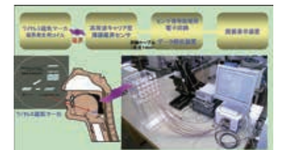
磁気式ワイヤレスモーションキャプチャ技術を用いた摂食嚥下機能評価システムの開発 Development of deglutition evaluation system using magnetic wireless motion capture system.
