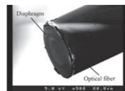
極細径光ファイバ圧力センサ(外径125 \mu m) Ultra-miniature fiber-optic pressure sensor (O.D. 125 \mu m)
