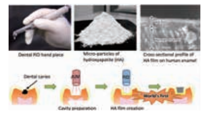
パウダージェットデポジション法を利用したハイドロキシアパタイト膜形成による革新的歯科治療法 New dental treatment utilizing powder jet deposition of hydroxyapatite
