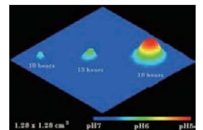
化学イメージングセンサによるpH分布の可視化 Visualization of pH by the chemical imaging sensor
