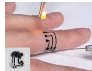
ハイドロゲル電極 Hydrogel-based microelectrodes
