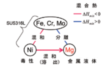
SUS316L表面から毒性ニッケル元素を脱成分する反応設計 Dealloying reaction design to remove toxic Ni element from SUS316L surface
