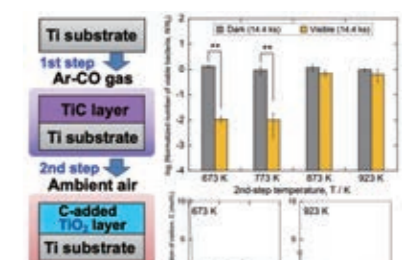
TiO 2 膜への可視光照射に伴う規格化細菌数の変化と含有される炭素濃度(可視光照射下で抗菌能を発現するアタナーゼ優位TiO 2 膜には炭素が含有されている、** p<0.01)
