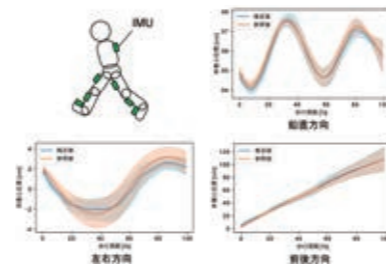
ウェアラブルセンサと機械学習を利用した歩行中の身体重心位置推定 Estimation of body center of mass position during gait using wearable sensors and machine learning
